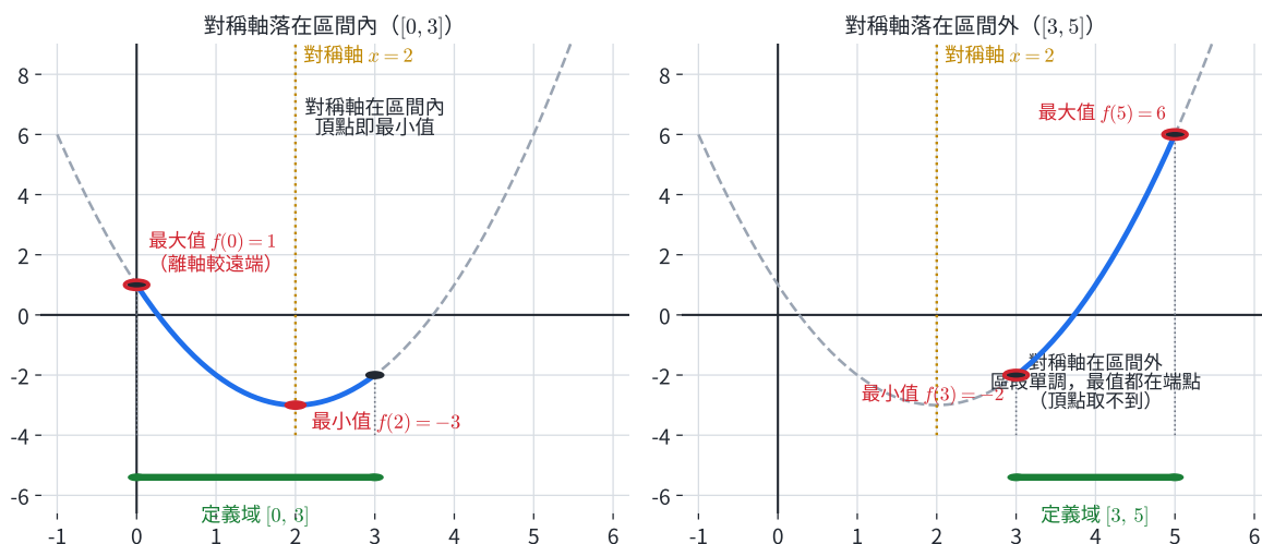
圖 2-2：閉區間上的二次極值，以 f(x) = (x - 2)^2 - 3 （頂點 (2, -3) 、開口向上）為例。左——定義域 [0, 3] ，對稱軸 x = 2 落在區間內，最小值在頂點 f(2) = -3 、最大值在離軸較遠的端點 f(0) = 1 。右——定義域 [3, 5] ，對稱軸落在區間外，區段單調遞增，最小、最大值都在端點 f(3) = -2 、 f(5) = 6 ，頂點取不到。粗藍線為定義域內的圖形，灰色虛線為區間外不計入的部分。
