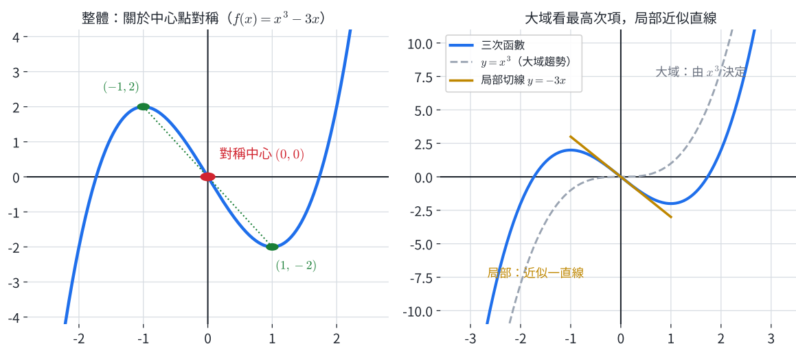
圖 2-4：左—— f(x) = x^3 - 3x 關於對稱中心 (0, 0) 點對稱：將點 (-1, 2) 與 (1, -2) 連線，中點即對稱中心。右——大域趨勢由最高次項 x^3 決定（兩端往相反方向延伸）；在對稱中心附近放大，曲線近似一條直線。
