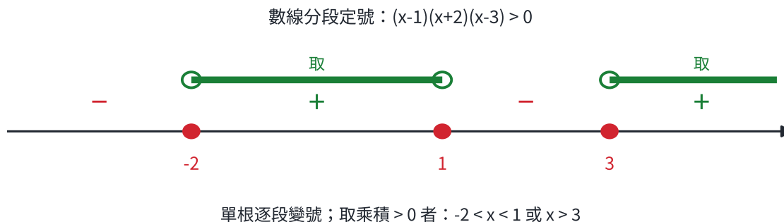
圖 2-6：數線分段定號，以 (x-1)(x+2)(x-3) > 0 為例。根 -2, 1, 3 把數線切成四段；最右段必為 + ，單根逐段交替為 -, +, -, + 。取乘積 > 0 的兩段（綠色，空心端點表示嚴格不等不含端點），解為 -2 < x < 1 或 x > 3 。
