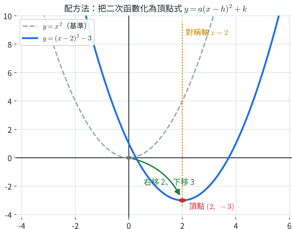
圖 2-3：以 y = (x - 2)^2 - 3 為例。把基準拋物線 y = x^2 （灰色虛線）右移 2、下移 3，得到頂點 (2, -3) 、對稱軸 x = 2 的拋物線（藍色實線）。
