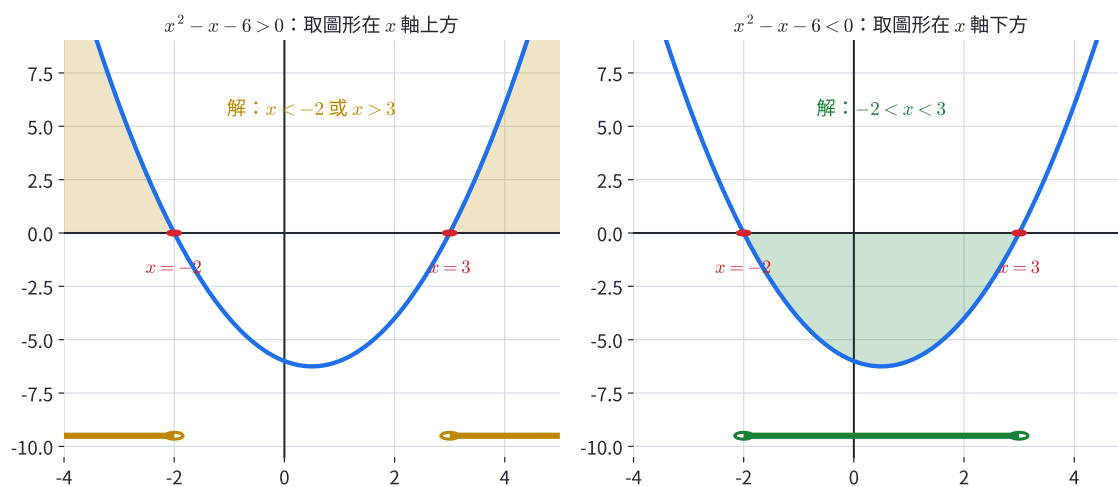
圖 2-5：以 x^2 - x - 6 = (x - 3)(x + 2) （根 -2, 3 ，開口向上）為例。左—— x^2 - x - 6 > 0 取圖形在 x 軸上方者，解為 x < -2 或 x > 3 （兩邊）；右—— x^2 - x - 6 < 0 取下方者，解為 -2 < x < 3 （中間）。
